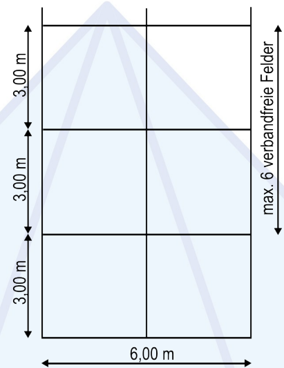
Draufsicht mit Bemaßungen
