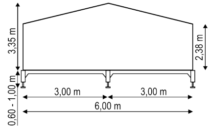
Seitenansicht mit Bemaßungen
