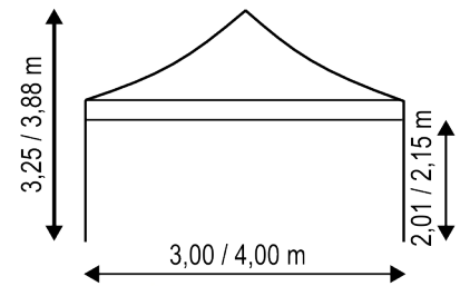
Seitenansicht der Quadratischen Zelte
