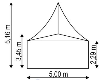
Seitenansicht mit Bemaßungen
