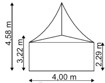
Seitenansicht mit Bemaßungen
